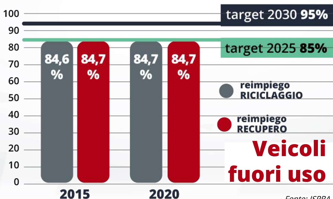
Tasso di impiego riciclo e tasso impiego recupero
