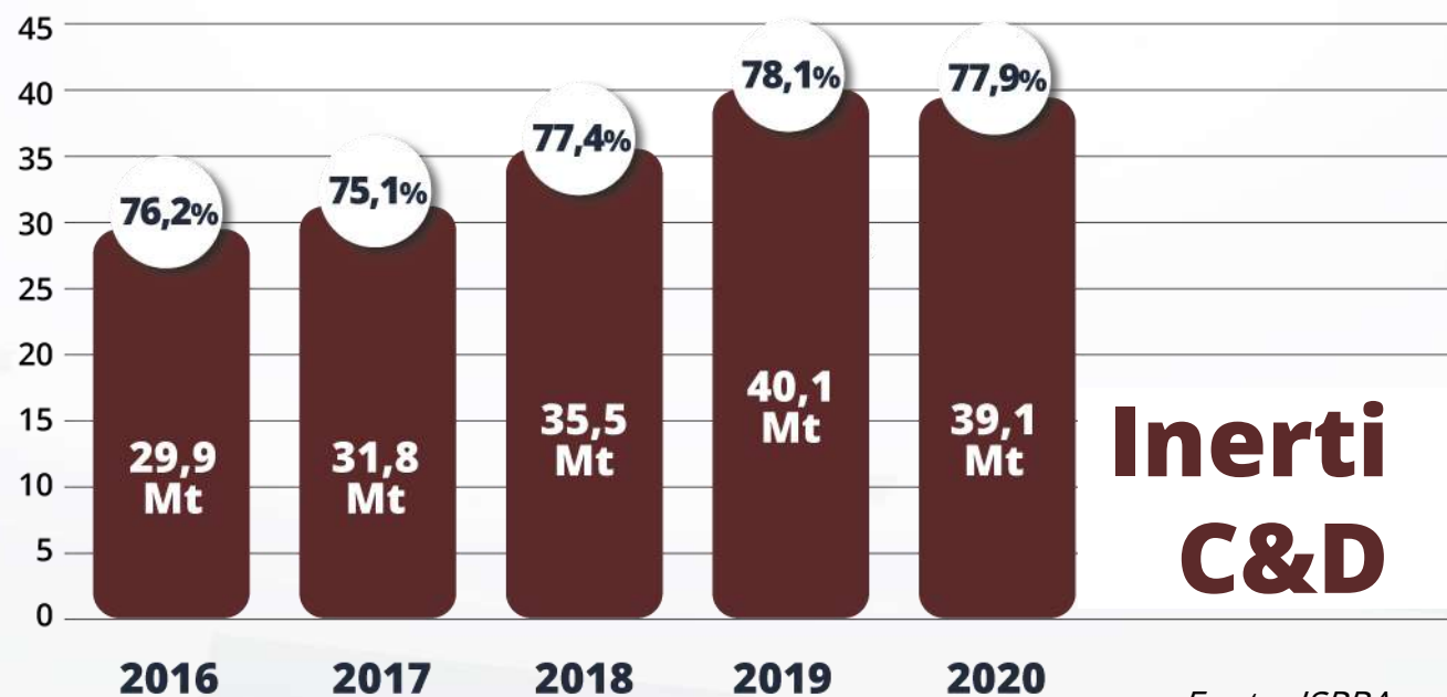
Quantità recuperate come materia dai rifiuti C&D (Mt) e andamento tasso recupero (%)
